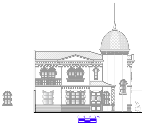
Elevation 01
